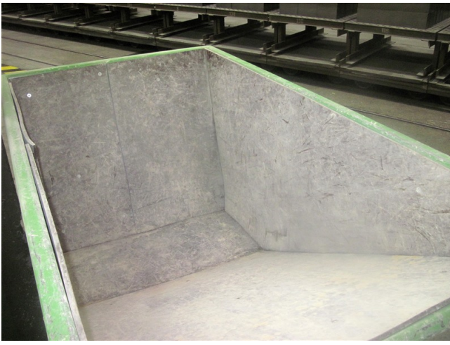
Gummiauskleidung der Kippkübel
