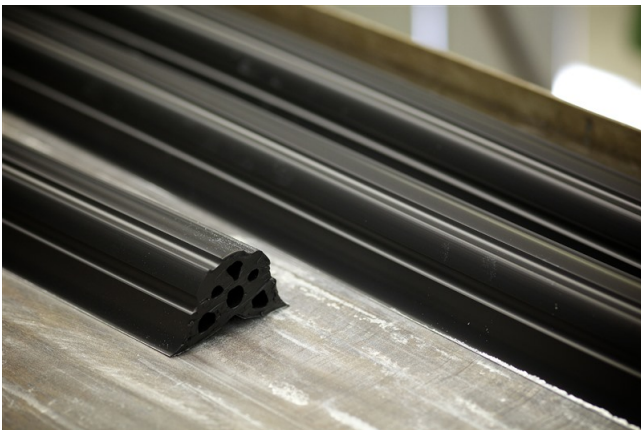
An den extrudierten Profilen kann man die Entwässerungskammern gut erkennen.
